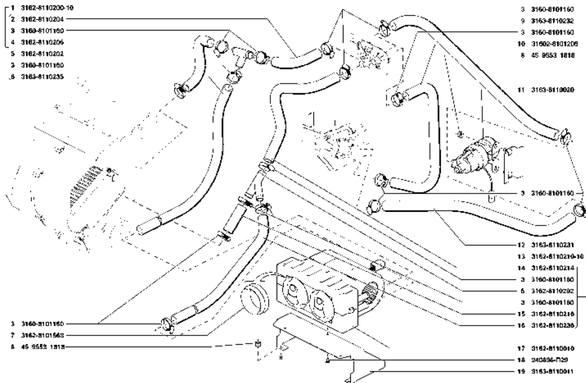
Рис. 120. Отопитель кузова задний (8110) Fig. 120. Body Rear Heater (8110)
