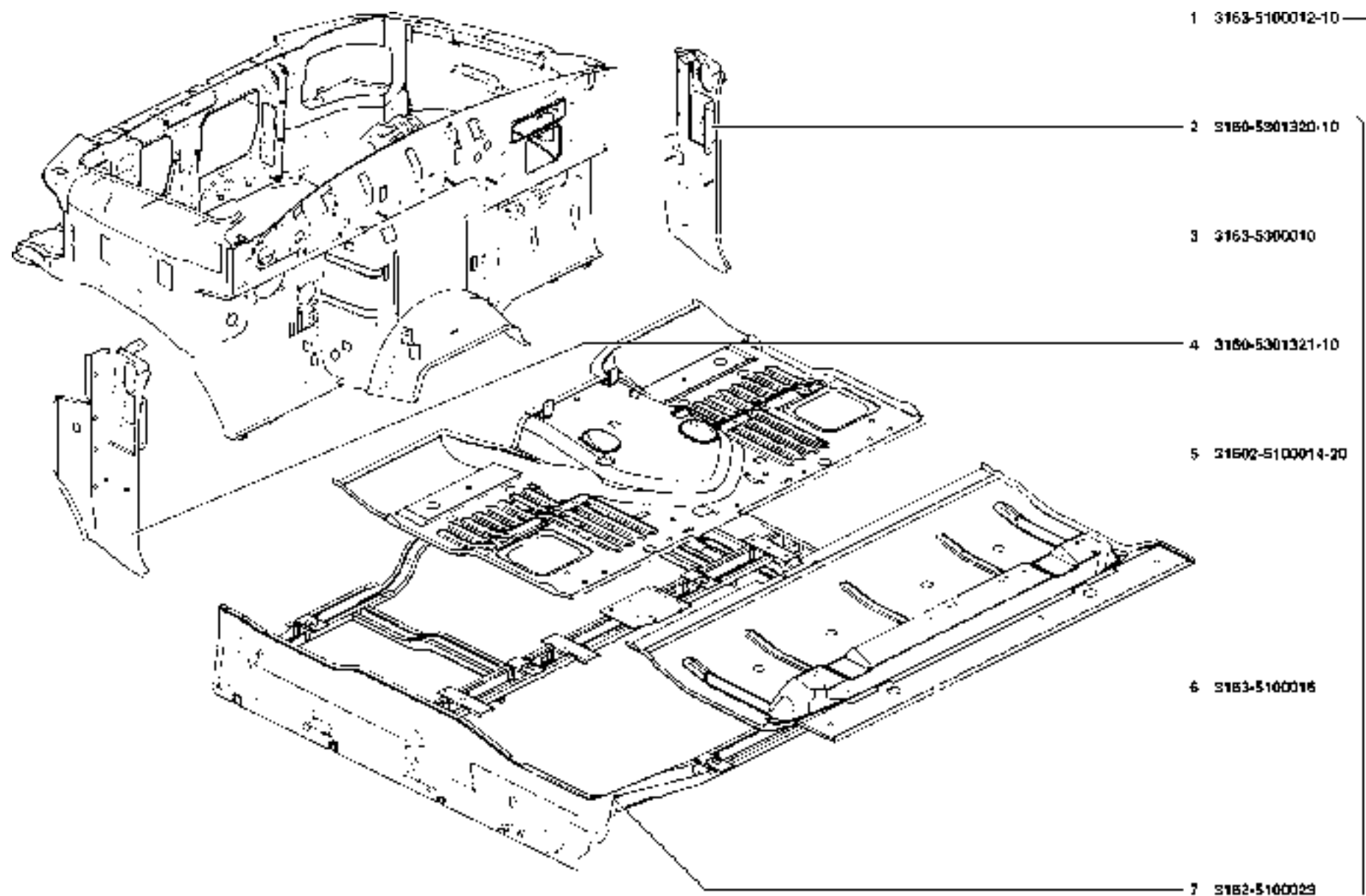
Рис. 95. Основание в сборе (5100)/1 Fig. 95. Base in Assy (5100)/1
