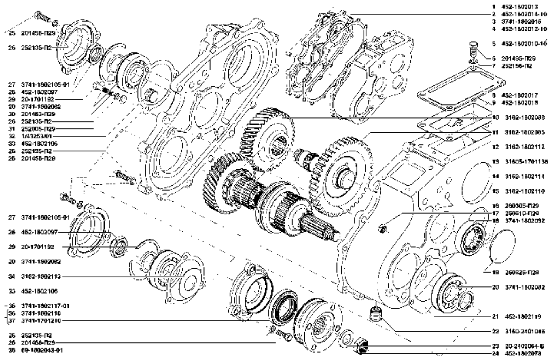
Рис. 35. Коробка раздаточная (1802)/1
