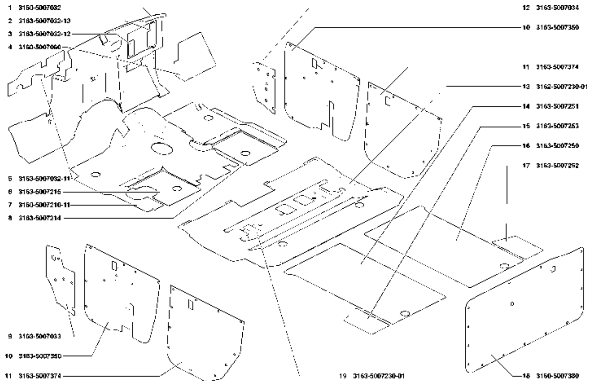
Рис. 94. Термозвукоизоляция кузова (5007) Fig. 94. Body Heat-And-Noise Insulation (5007)
