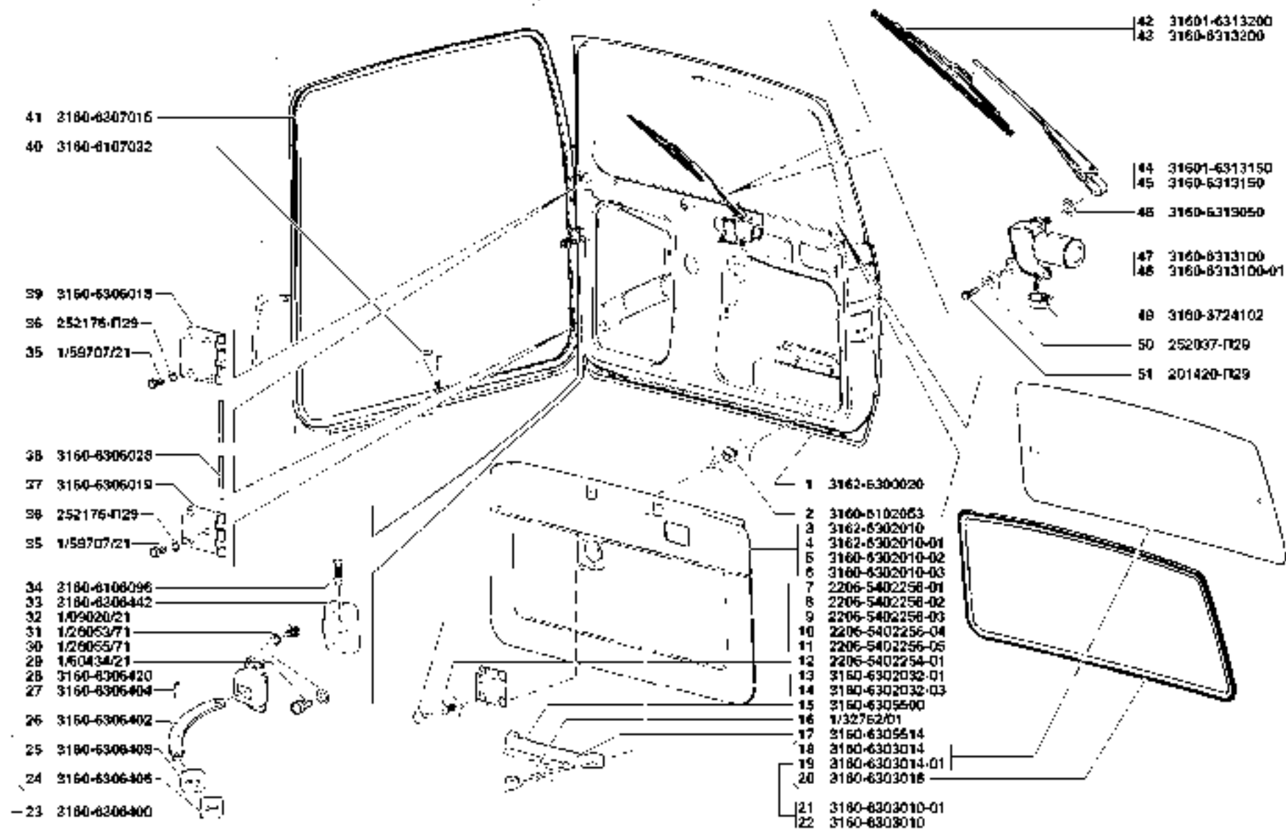
Рис. 122. Зеркала (8201), поручни, крючки для одежды (8202), пепельница (8203), козырьки противосолнечные (8204)
