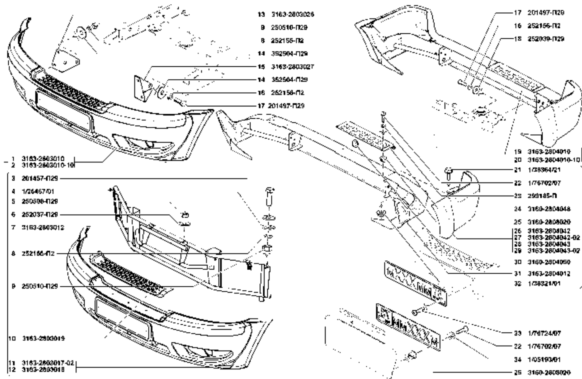
Рис. 49. Бампер передний (2803), бампер задний (2804), крепление переднего номерного знака (2807) и крепление заднего номерного знака (2808) Fig. 49. Front Bumper (2803), Rear Bumper (2804), Front Licence Plate Attaching Parts (2807) And Rear Licence Plate Attaching Parts (2808)
