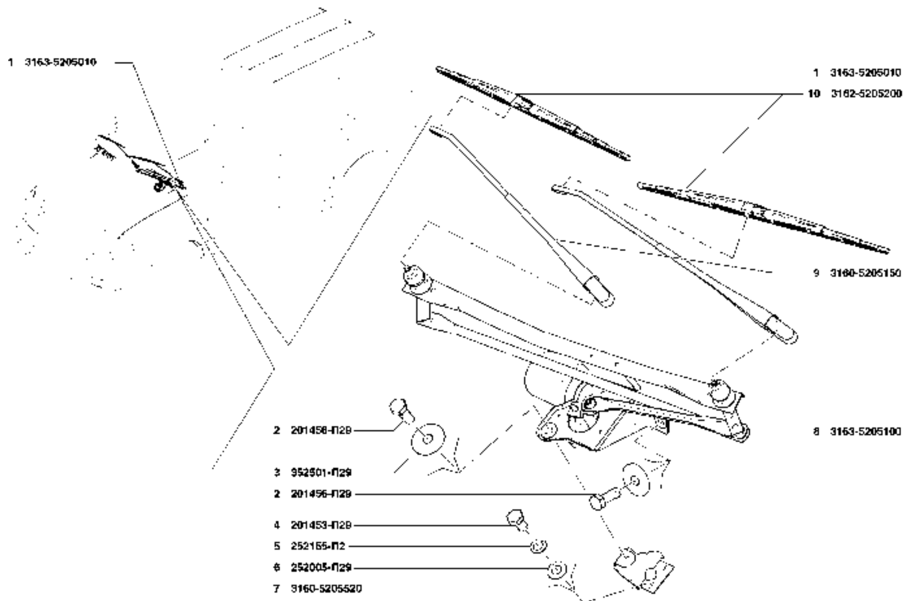
Рис. 100. Стеклоочиститель и привод (5205) Fig. 100. Windshield Wiper and Drive (5205)
