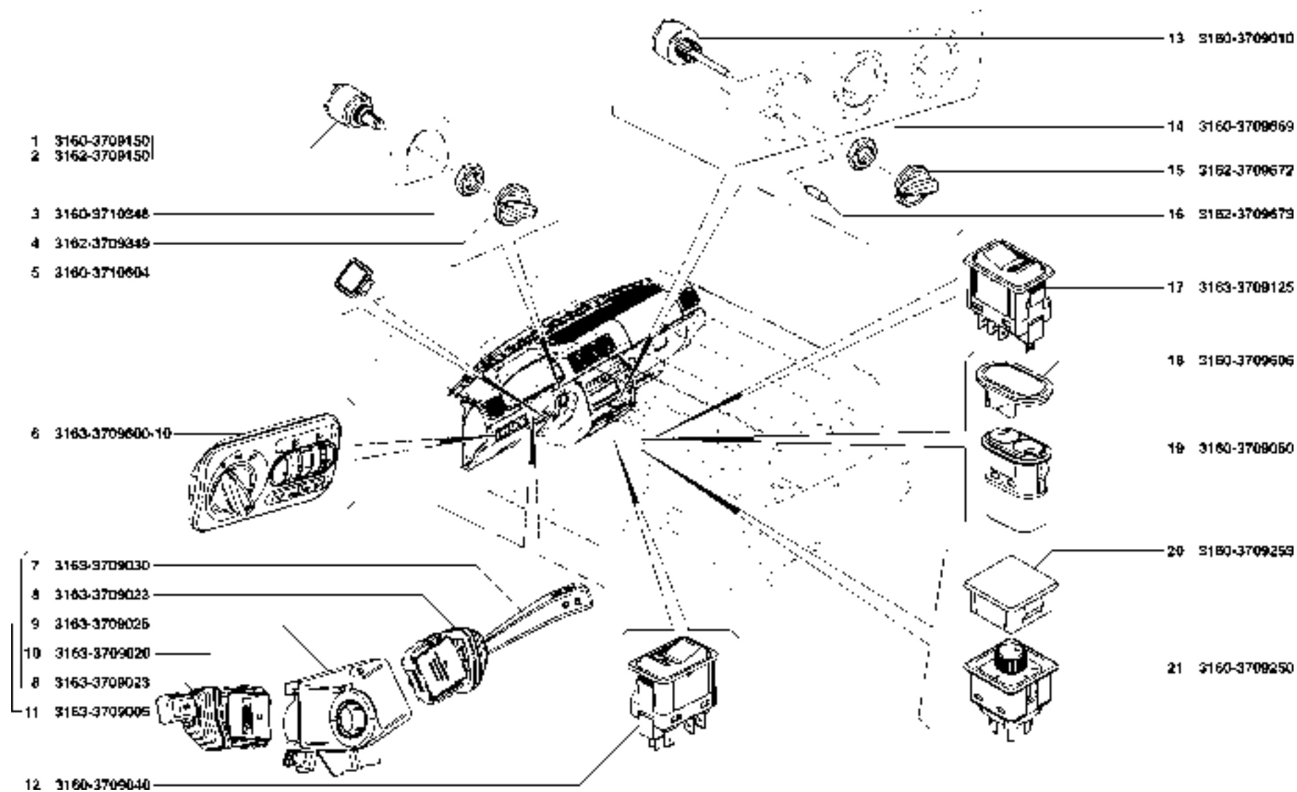
Рис. 76. Переключатели (3709) Fig. 76. Selector Switches (3709)
