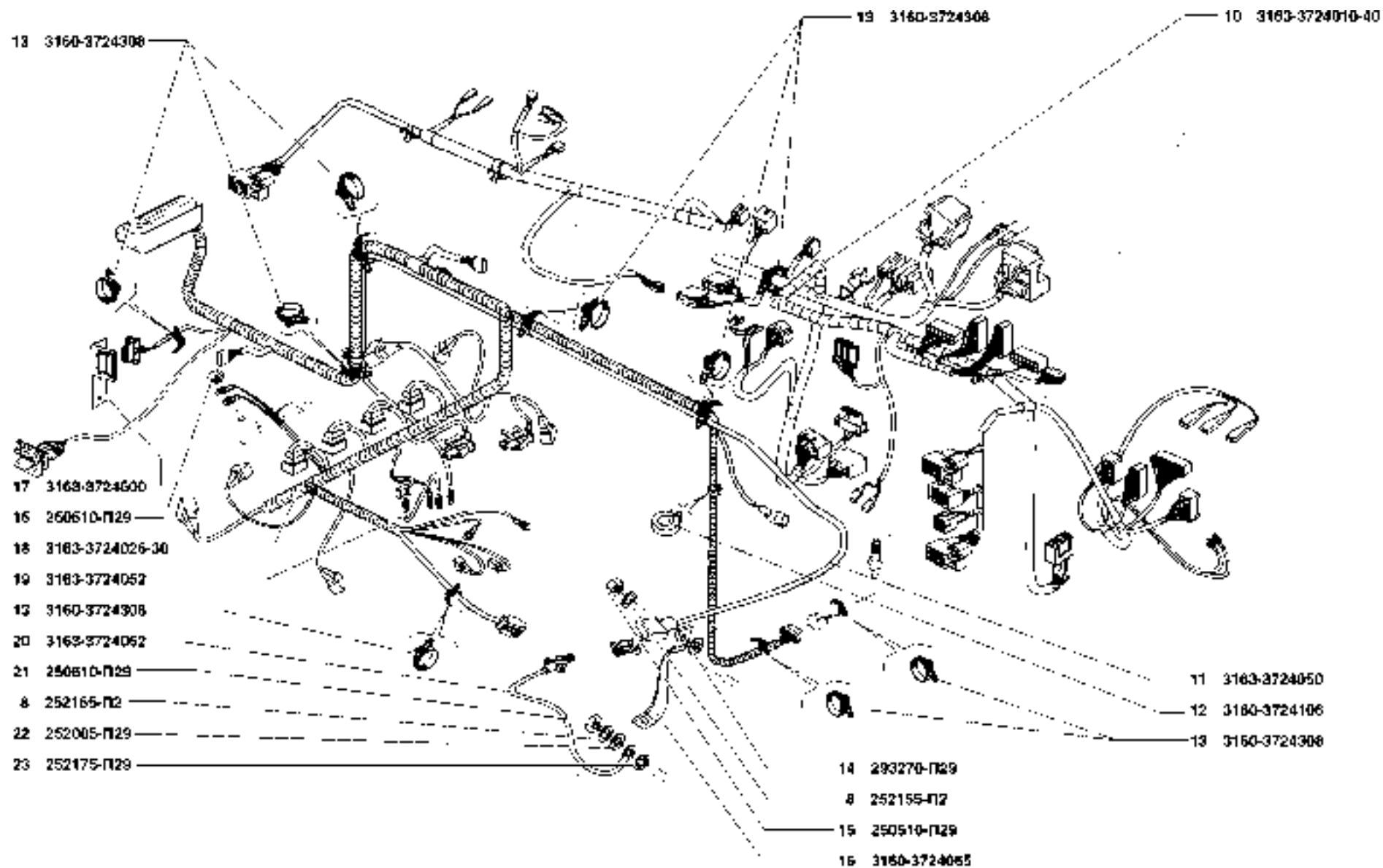
Рис. 82. Электропровода (3724)/2 Fig. 82. Wires (3724)/2
