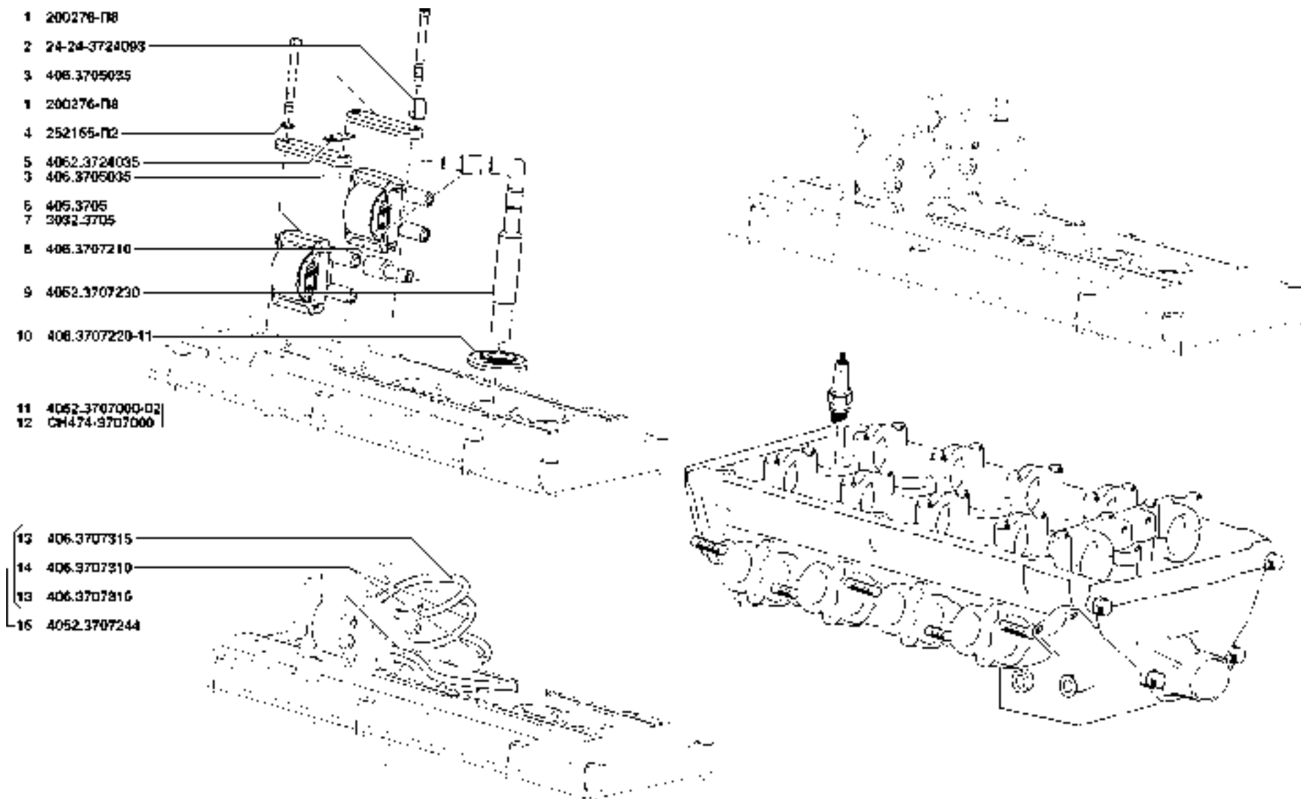
Рис. 74. Катушка зажигания (3705), свечи и провода зажигания (3707) Fig. 74. Ignition Coil (3705), Ignition Plugs and Wires (3707)
