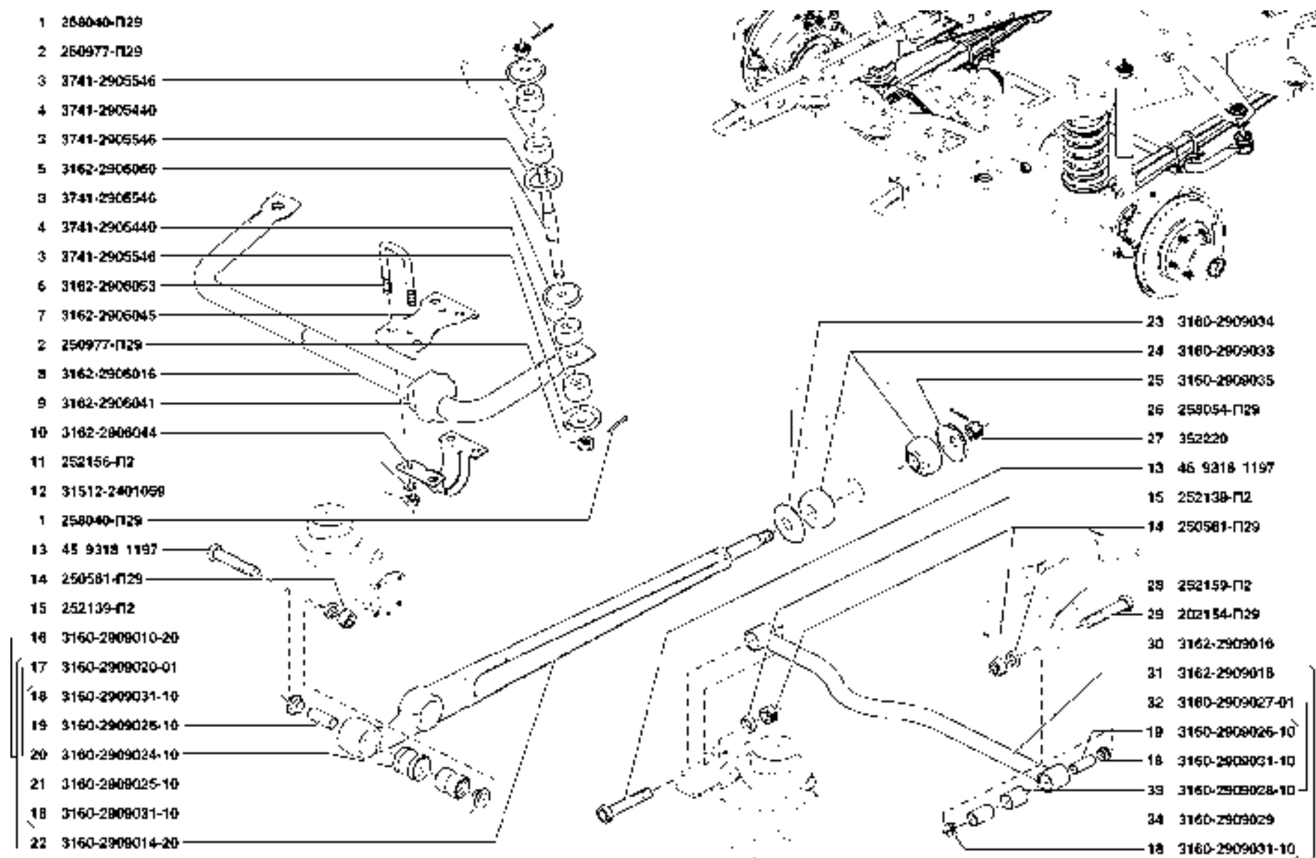
Рис. 51. Стабилизатор поперечной устойчивости (2906), штанги реактивные передней подвески (2909)
