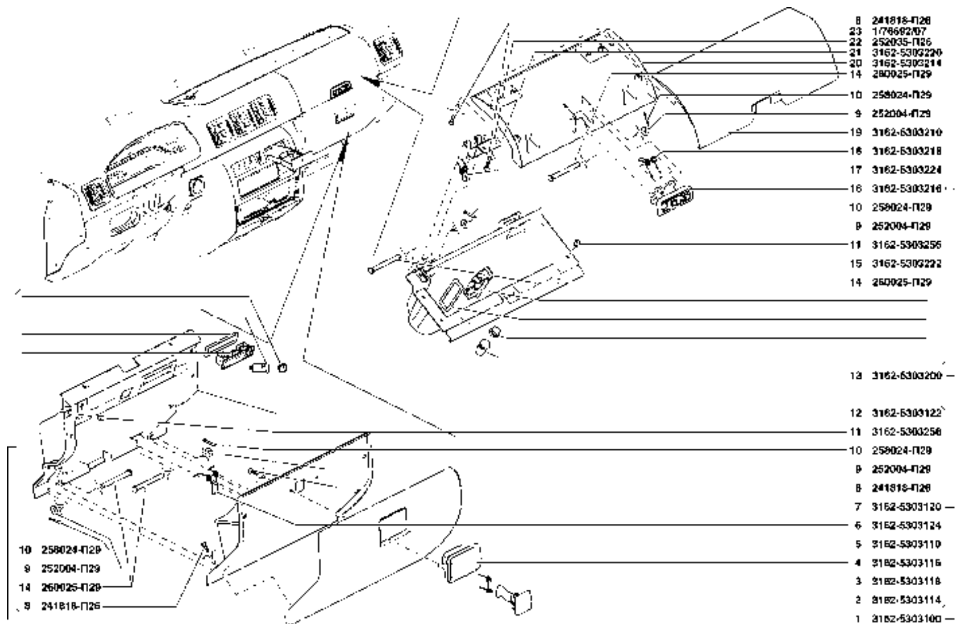
Рис. 102. Ящик вещевой (5303) Fig. 102. Glove Box (5303)
