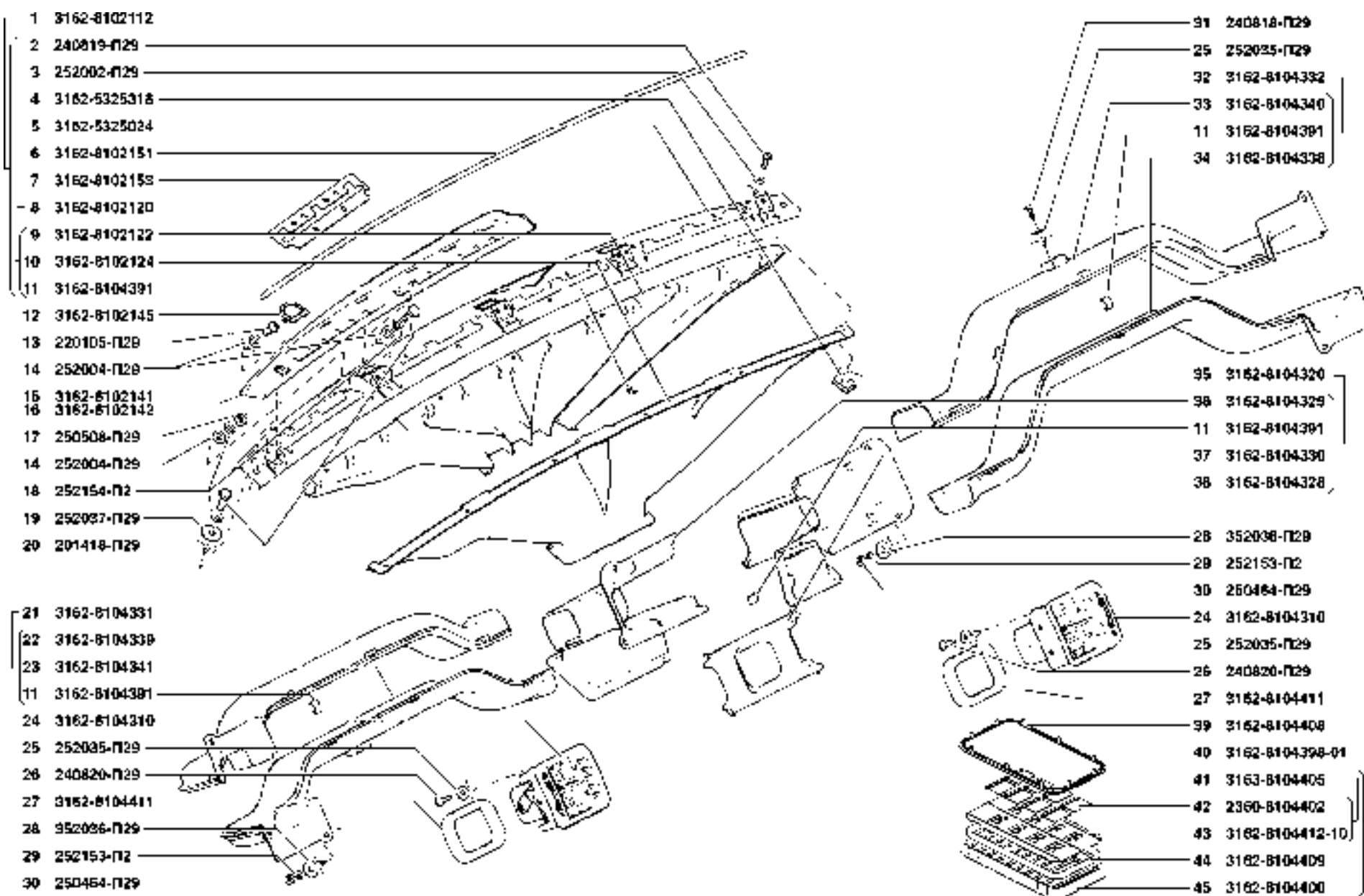
Рис. 118. Обогрев ветрового стекла (8102), вентиляция кузова (8104) Fig. 118. Windshield Hot-Air Defroster (8102), Body Ventilation (8104)
