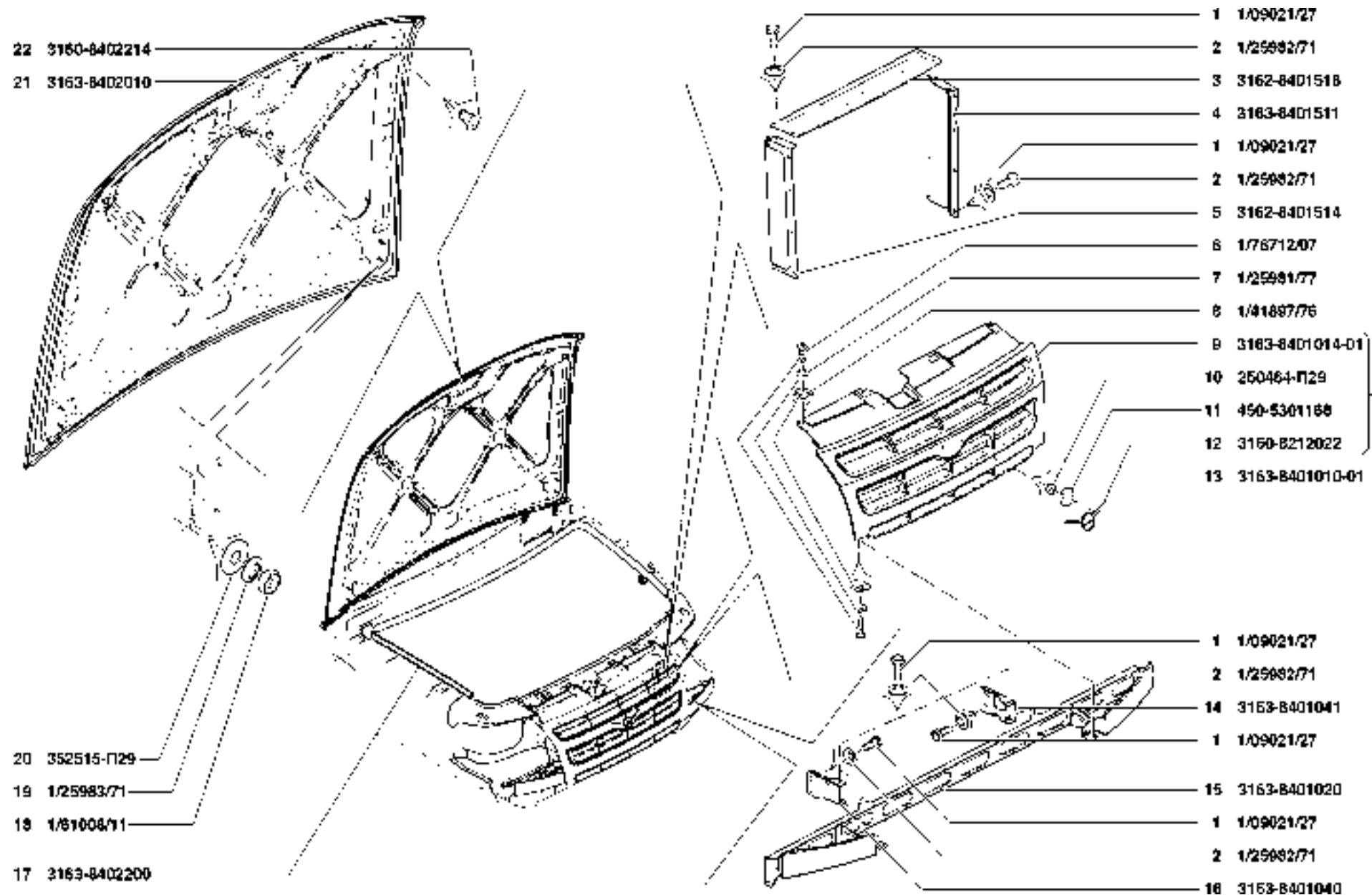
Рис. 125. Облицовка радиатора (8401), капот (8402) Fig. 125. Radiator Grille (8401), Hood (8402)
