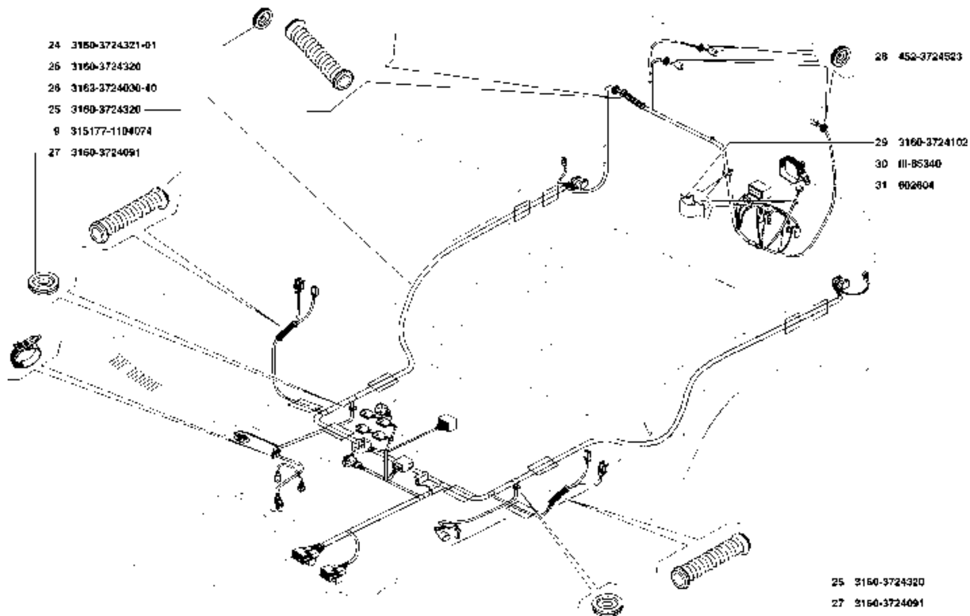
Рис. 83. Электропровода (3724)/3 Fig. 83. Wires (3724)/3
