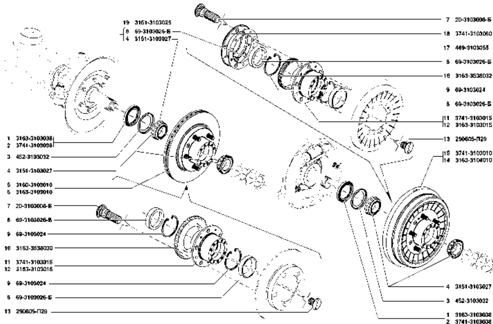
Рис. 55. Ступицы передних и задних колес (3103) Fig. 55. Front And Rear Wheel Hubs (3103)
