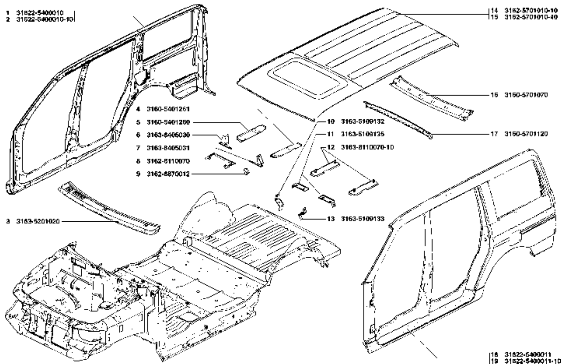
Рис. 92. Кузов в сборе (5000) Fig. 92. Body Assy (5000)
