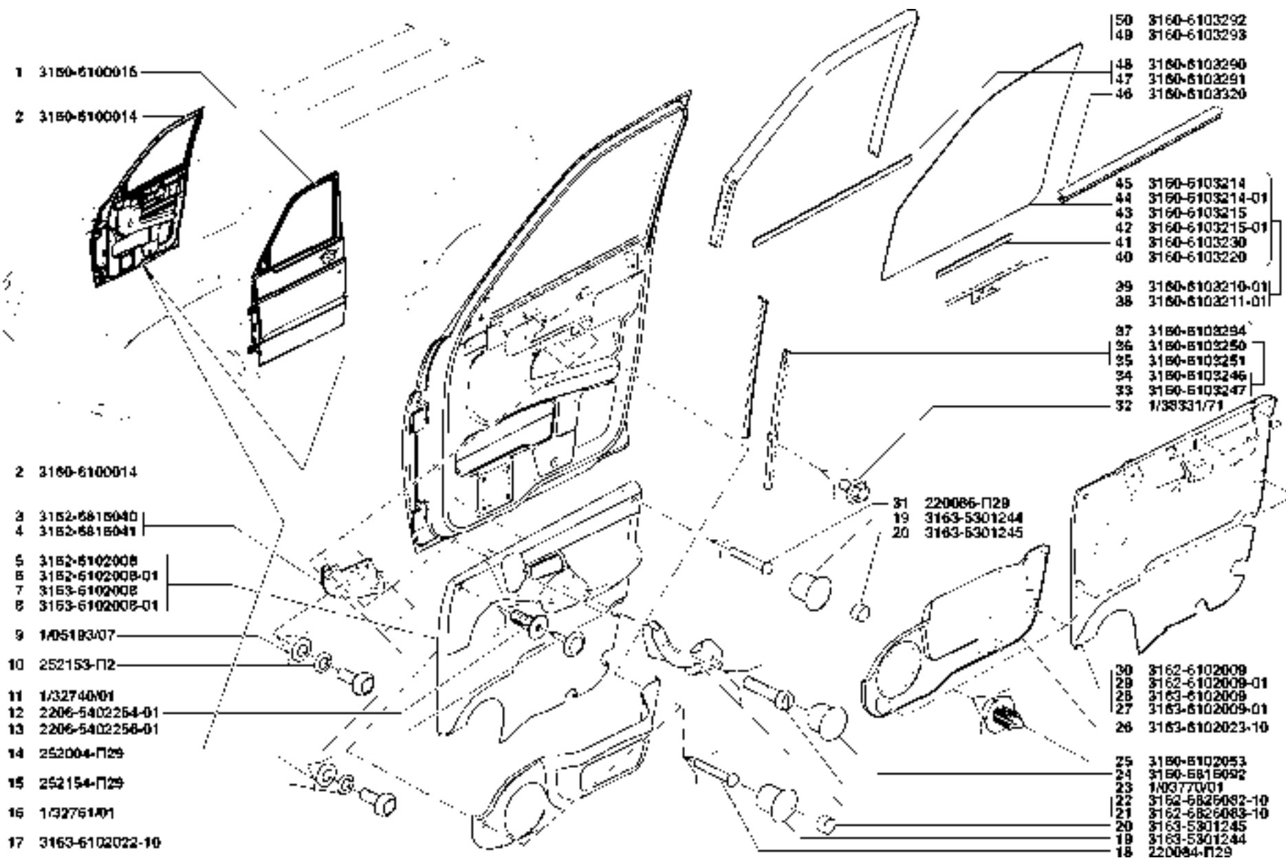
Рис. 107. Дверь передняя в сборе (6100), обивка передней двери (6102), окно передней двери (6103)
