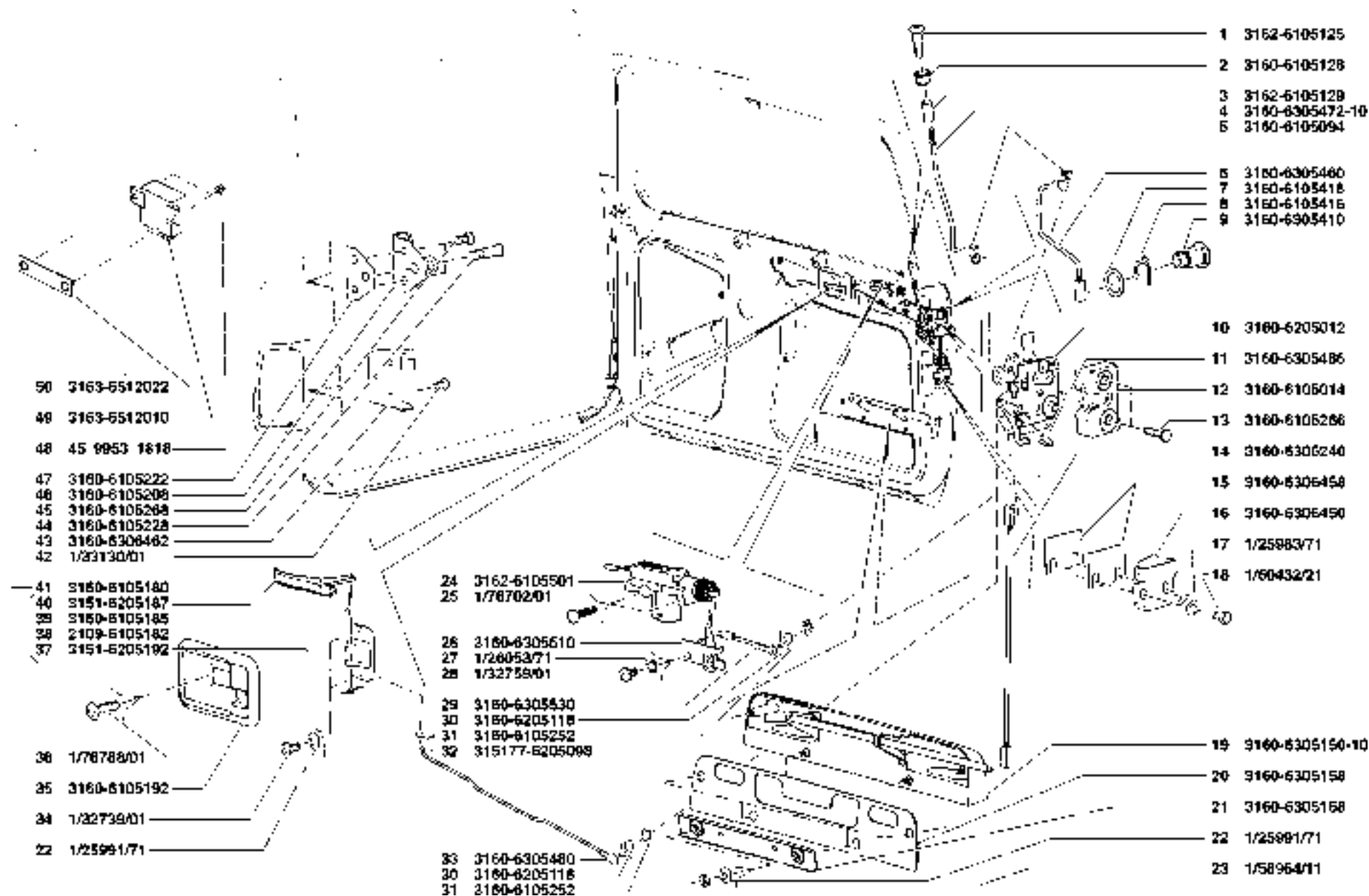
Рис. 114. Замок и ручки двери задка (6305), блок электронный управления электроблокировкой замков двери и исполнительные органы (6512)
