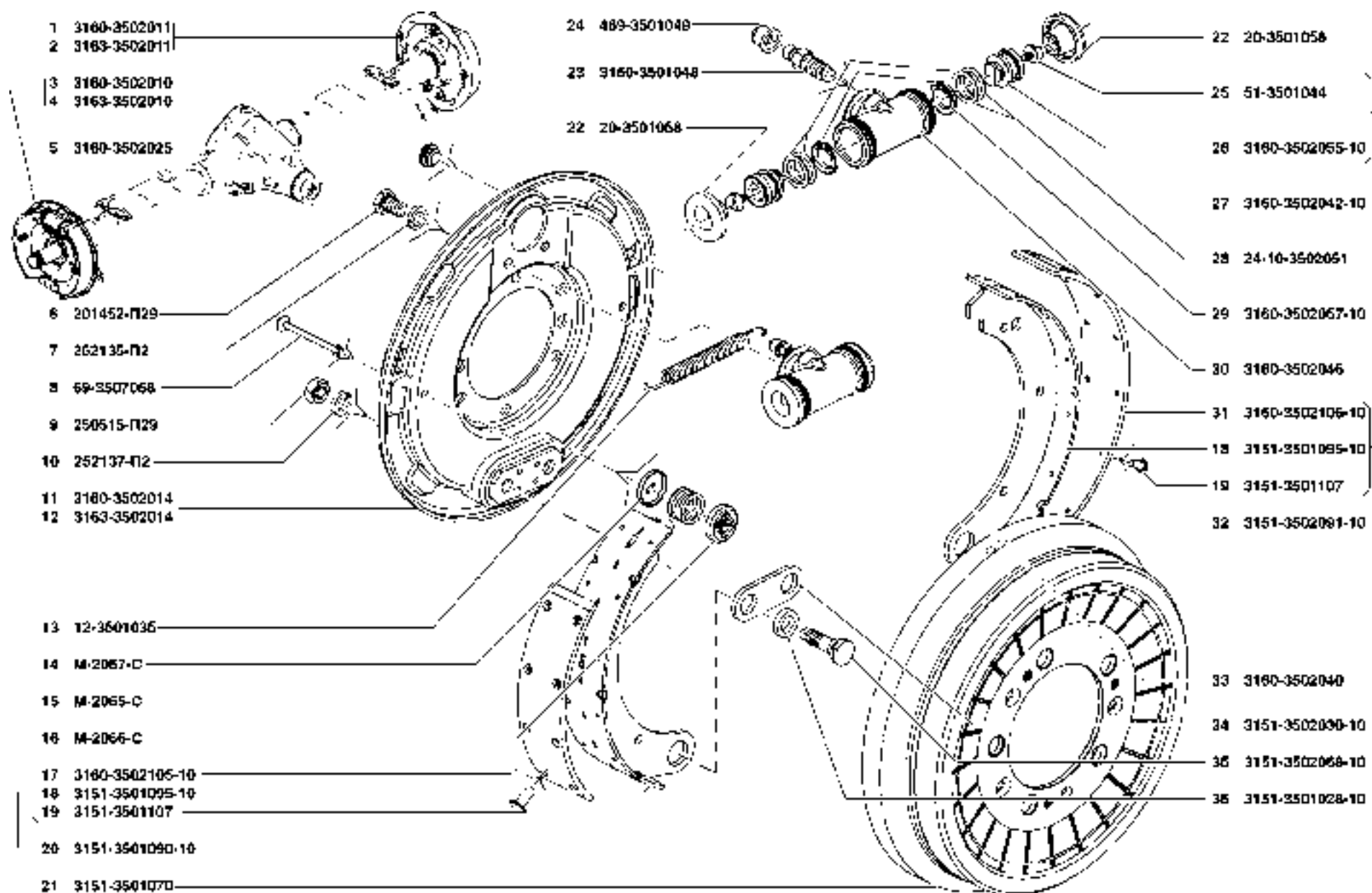
Рис. 63. Тормоза рабочие задние и тормозные барабаны (3502)
