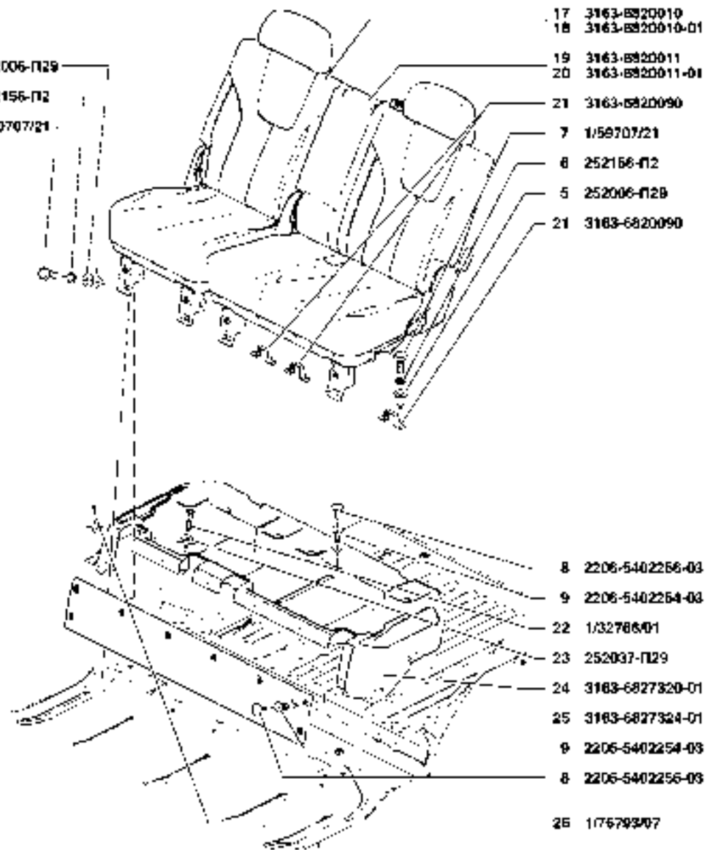
Рис. 115. Сиденье переднее (6810), сиденье заднее (6820) Fig. 115. Front Seat (6810), Rear Seat (6820)
