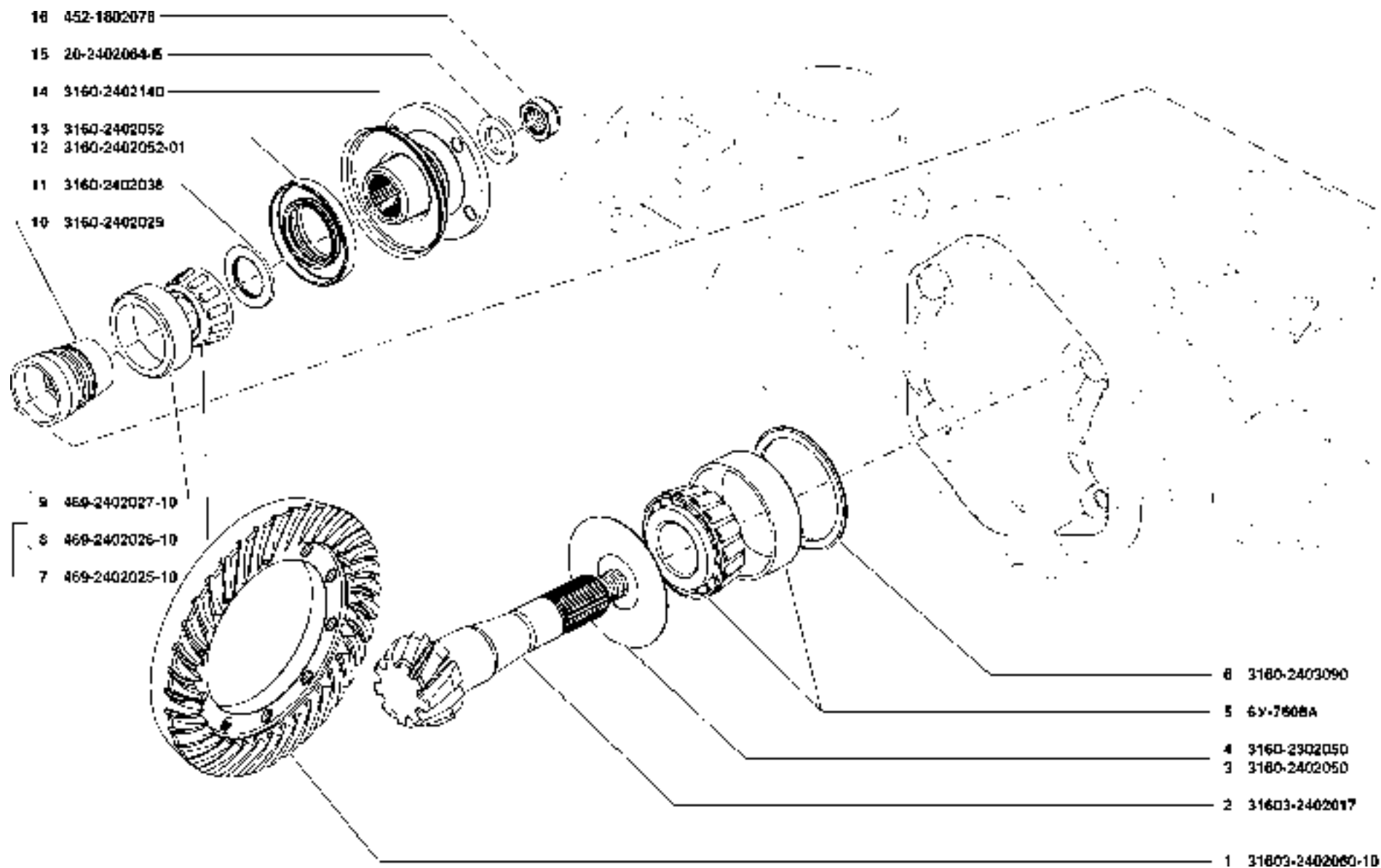
Рис. 46. Передача главная переднего и заднего мостов (2402) Fig. 46. Front And Rear Axle Final Drive (2402)
