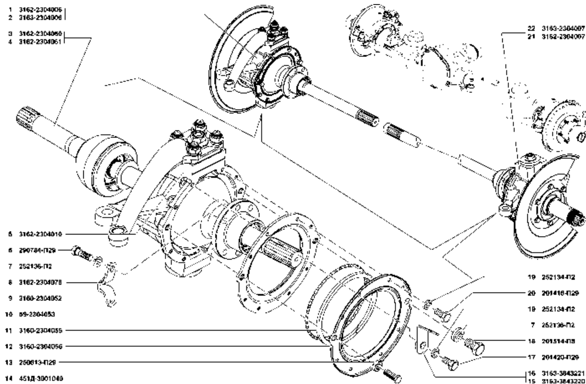
Рис. 42. Кулаки поворотные (2304)/1 Fig. 42. Steering Knuckles (2304)/1
