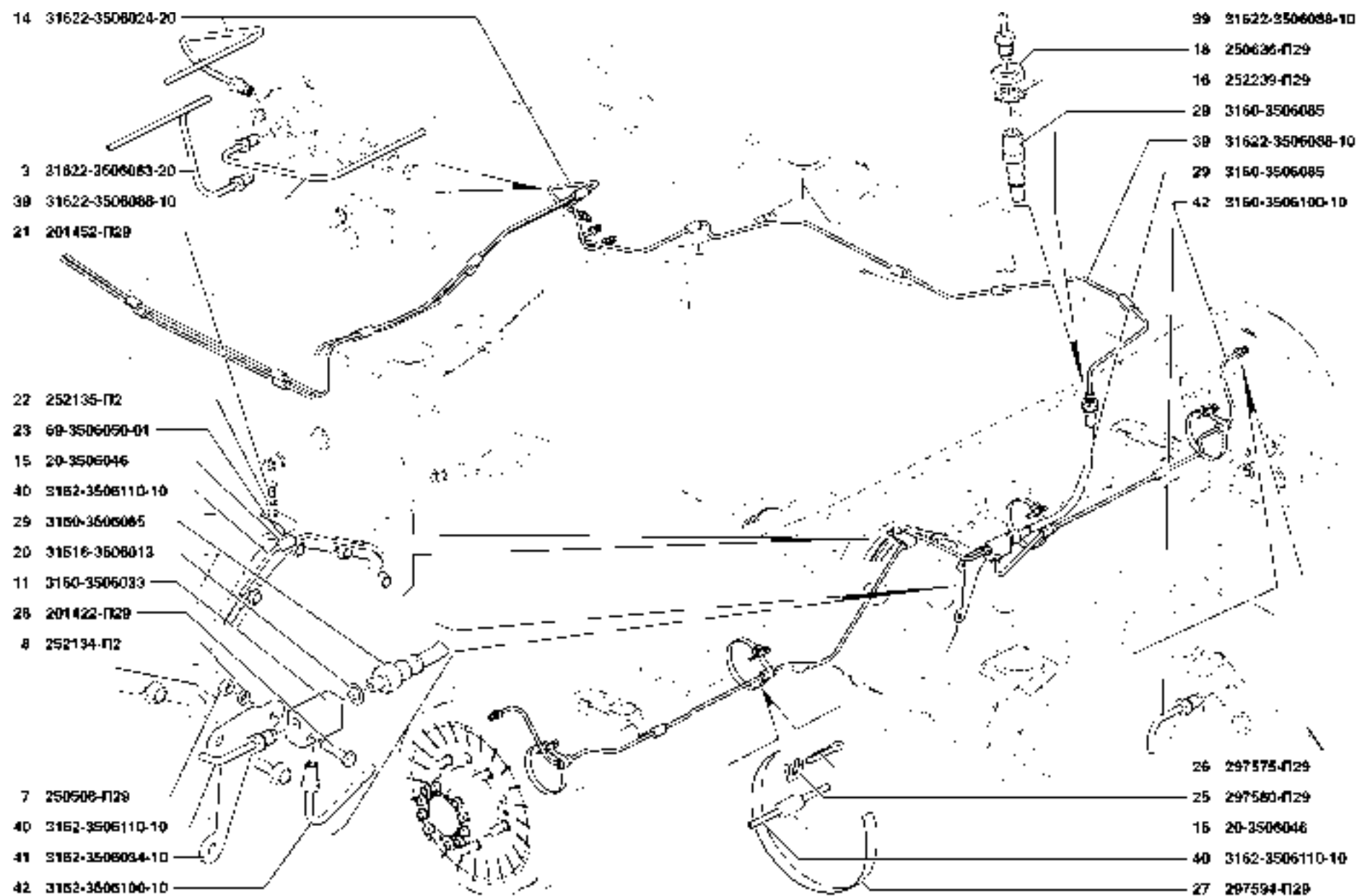
Рис. 67. Трубопроводы гидротормозов (3506)/3 Fig. 67. Hydraulic Brake Pipes (3506)/3
