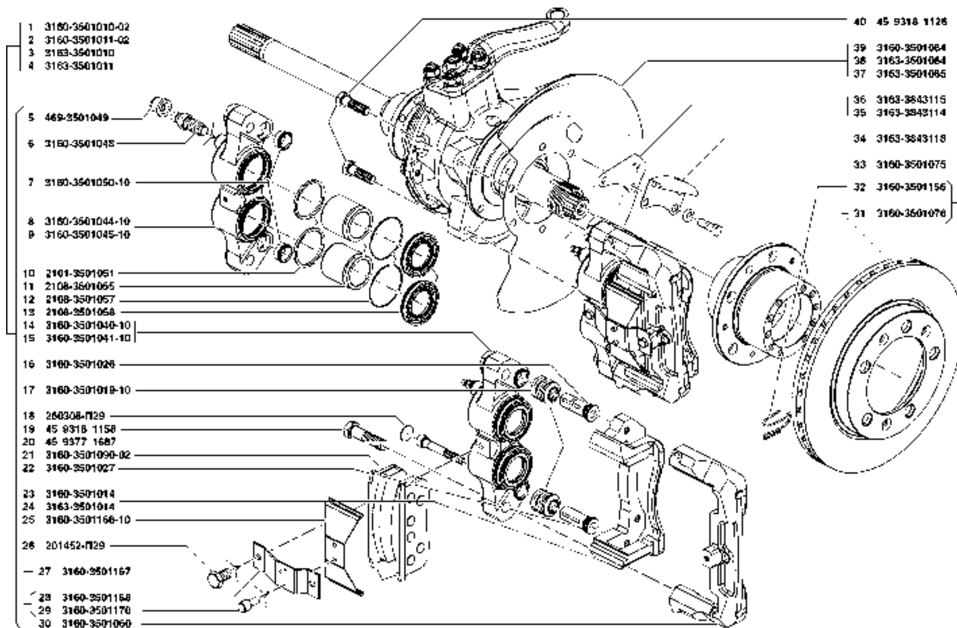
Рис. 62. Тормоза рабочие передние и тормозные диски(3501) Fig. 62. Front Wheel Service Brakes and Brake Disks (3501)
