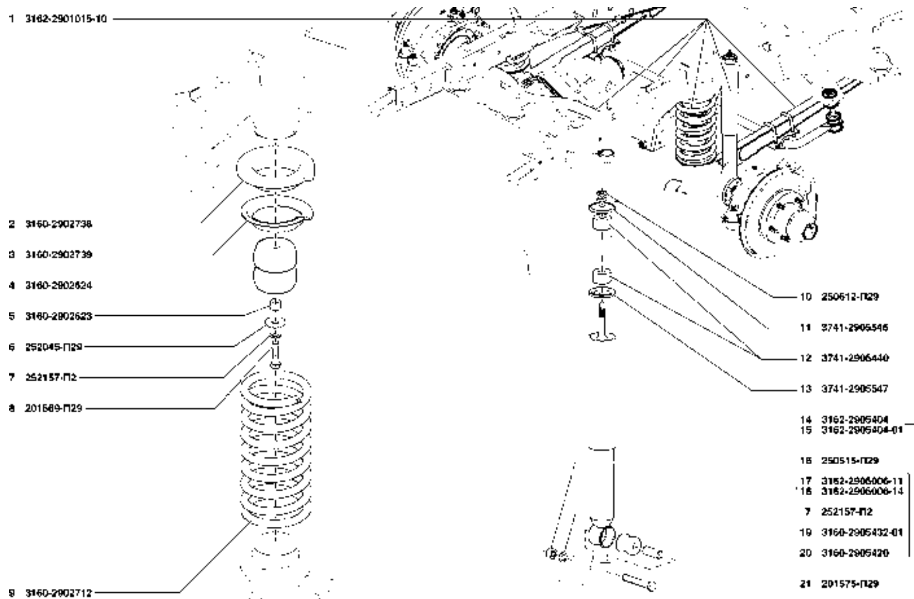
Рис. 50. Подвеска передняя в сборе (2901), пружины передние (2902), амортизаторы передние (2905) Fig. 50. Front Suspension In Assy (2901), Front Springs (2902), Front Shock Absorbers (2905)
