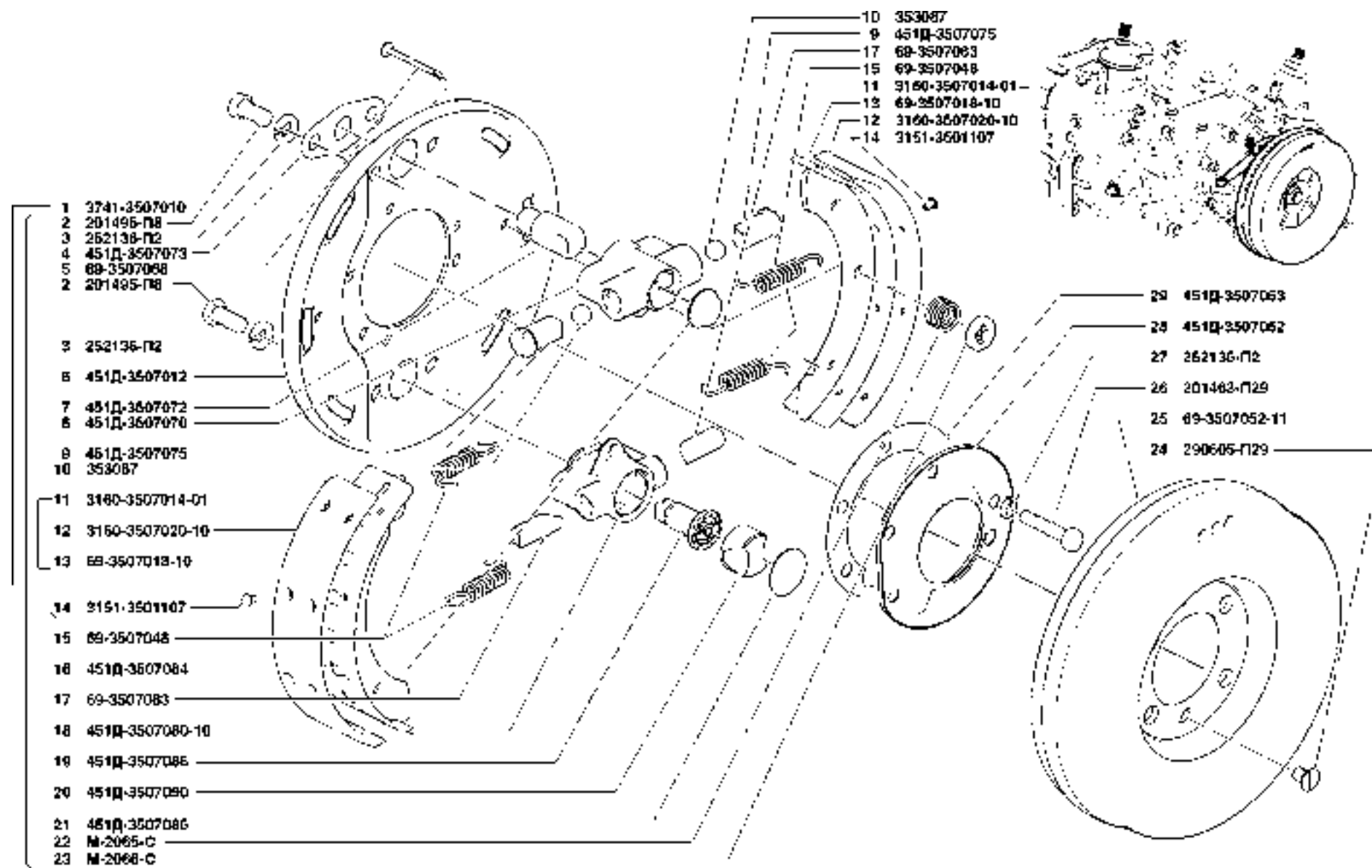
Рис. 69. Стояночный тормоз (3507)
