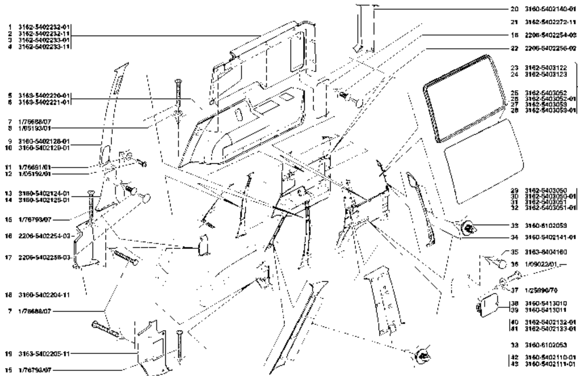
Рис. 105. Обивка боковины (5402), окно боковины (5403), люк боковины (5413)
