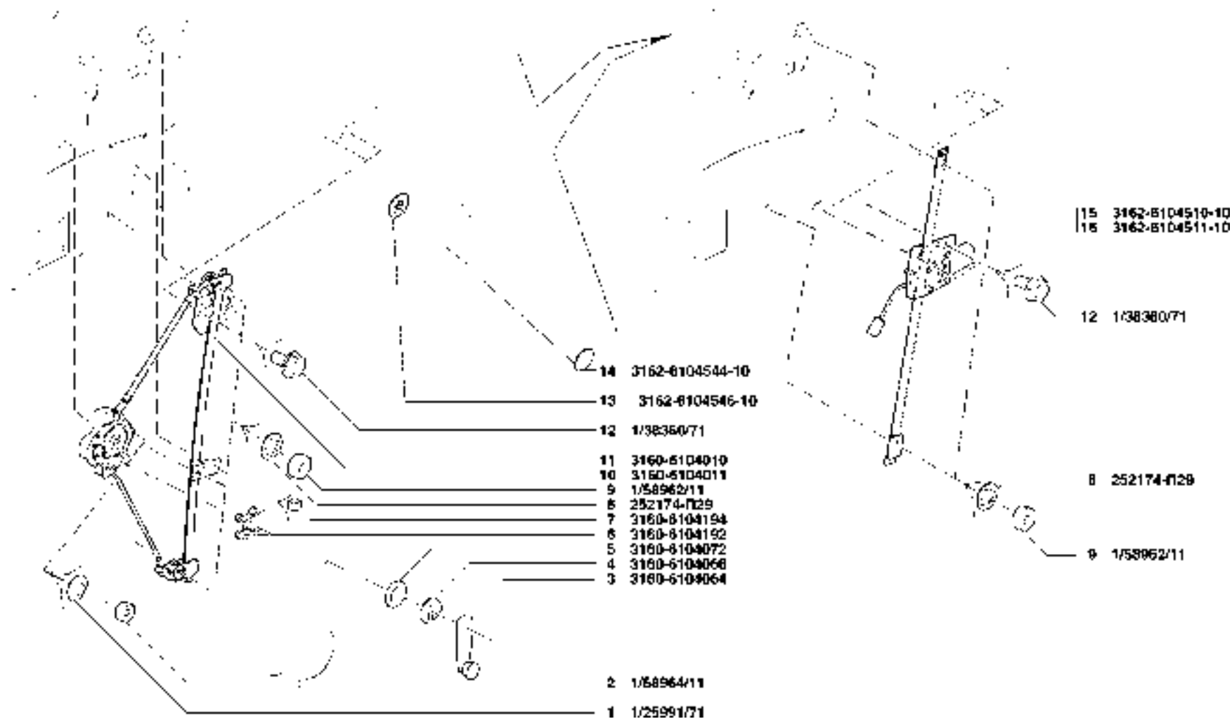
Рис. 108. Механизм перемещения стекла передней двери (6104) Fig. 108. Front Door Glass Shifting Mechanism (6104)
