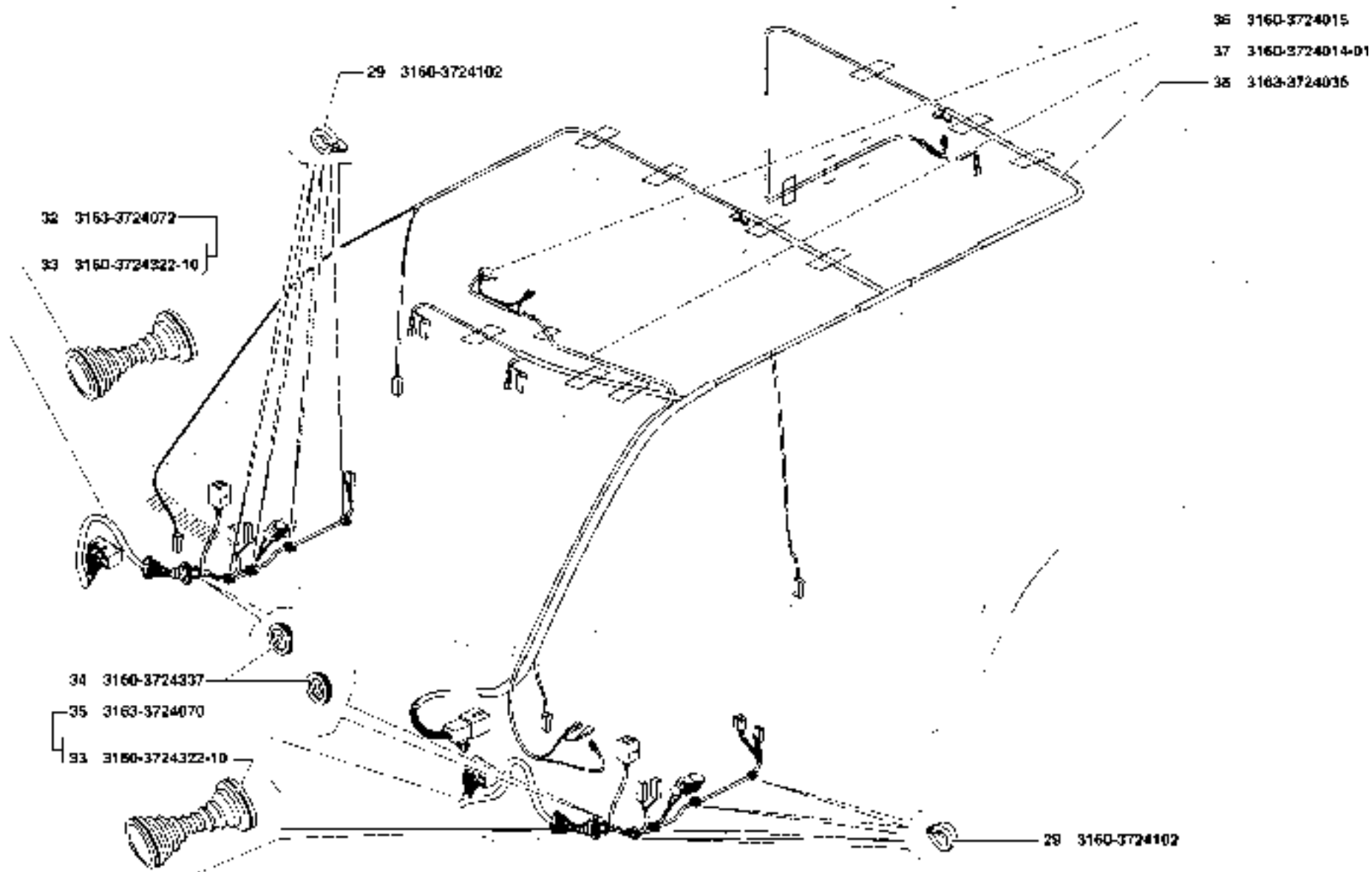
Рис. 84. Электропровода (3724)/4 Fig. 84. Wires (3724)/4
