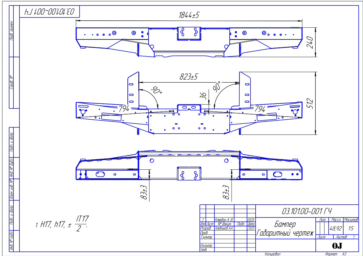
Рис. 3. Габаритный чертёж.
